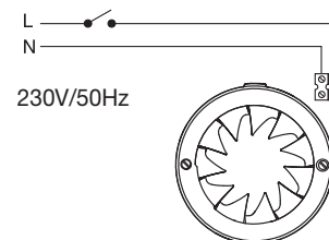
připojení ventilátoru k síti
