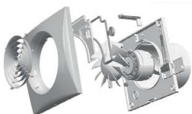
konstrukce ventilátoru
