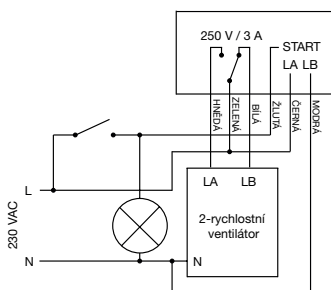
DT 3-PR po sejmutí krytu
